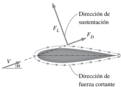
FIGURA 11-40 Para las superficies de sustentación, la aportación de los efectos viscosos es despreciable, por lo general, porque la fuerza cortante es paralela a la superficie y por lo tanto casi normal a la dirección de sustentación.
