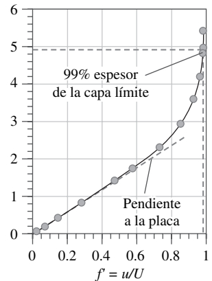
FIGURA 10-99 Perfil de Blasius en variables de similitud para la capa límite que crece sobre una placa plana semiinfinita. Los datos experimentales (círculos) son a \text{Re}_x = 3.64 \times 10^5 . Tomado de Panton (1996).
