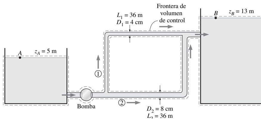
FIGURA 8-47 Sistema de tuberías comentado en el Ejemplo 8-7.
