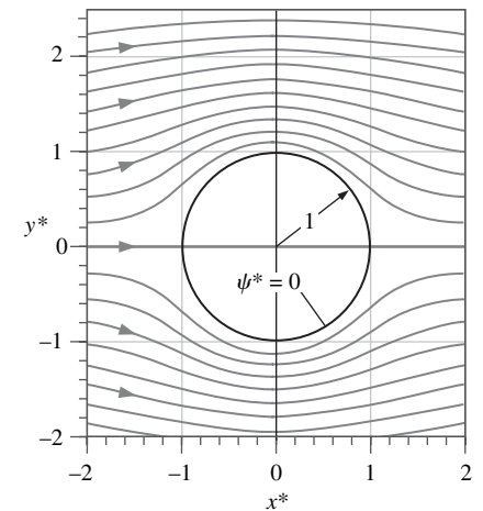
FIGURA 10-61 Líneas de corriente adimensionales creadas por superposición de un flujo uniforme y un doblete en el origen \psi^* = \psi/(V_\infty a) , \Delta \psi^* = 0.2 , x^* = x/a , y y^* = y/a , donde a es el radio del cilindro.
