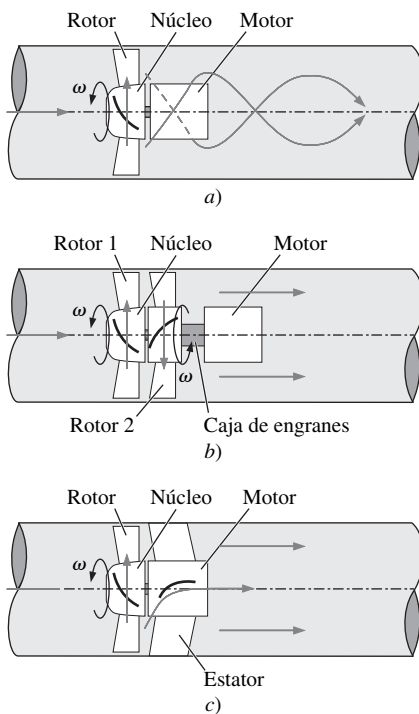
FIGURA 14-57 Un ventilador de flujo axial entubado a) impone el movimiento giratorio al flujo existente, mientras que b) un ventilador de flujo axial con el segundo rotor contrarrotatorio y c) un ventilador de flujo axial con el estator de álabes guía están diseñados para eliminar el movimiento giratorio.
