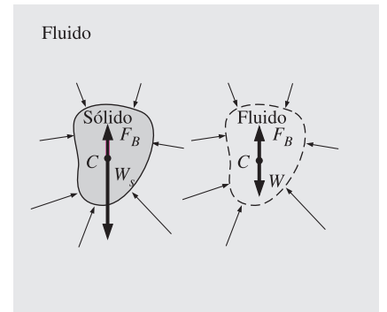
FIGURA 3-38 Las fuerzas de flotación que actúan sobre un cuerpo sólido sumergido en un fluido y sobre una masa del fluido de la misma forma, a la misma profundidad, son idénticas. La fuerza de flotación F_B actúa hacia arriba pasando por el centroide C del volumen desplazado y es igual en magnitud al peso W del fluido desplazado, pero en la dirección opuesta. Para un sólido de densidad uniforme, su peso W_s también actúa pasando por el centroide, pero su magnitud no es necesariamente igual a la del fluido que desplaza. (Aquí, W_s > W y, donde W_s > F_B , este cuerpo sólido se hundiría.)
