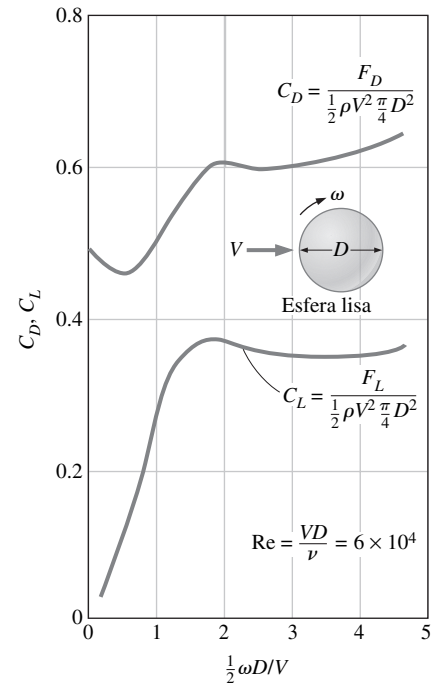
FIGURA 11-53 Variación de los coeficientes de sustentación y de arrastre de una esfera lisa con la razón de rotación adimensional para Re = VD/\nu = 6 \times 10^4 . Tomado de Goldstein, 1938.
