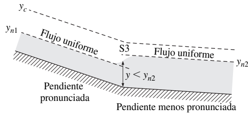
c) Flujo uniforme supercrítico que cambia desde una pendiente pronunciada a la pendiente menos pronunciada
