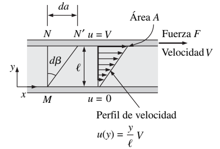
FIGURA 2-12 Comportamiento de un fluido en flujo laminar entre dos placas paralelas, cuando la placa superior se mueve con una velocidad constante.
