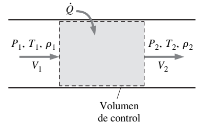
FIGURA 12-51 Volumen de control para el flujo en un ducto de área constante con transferencia de calor y de fricción despreciable.
