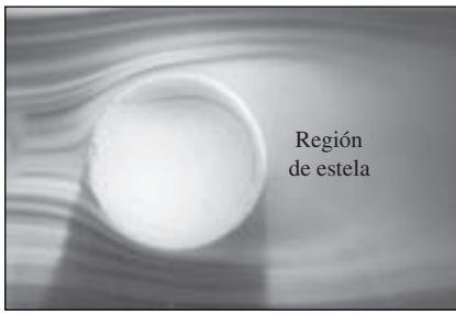
FIGURA 11-15 Separación de flujo sobre una pelota de tenis y la región de estela. Cortesía de NASA y Cislunar Aerospace, Inc.
