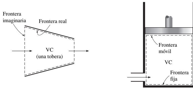
a) Un volumen de control (VC) con fronteras real e imaginaria
