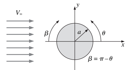
FIGURA 10-62 Flujo planar sobre un cilindro circular de radio a que está sumergido en un flujo uniforme de velocidad V_\infty en el plano xy . Por costumbre, el ángulo \beta se define desde el frente del cilindro.
