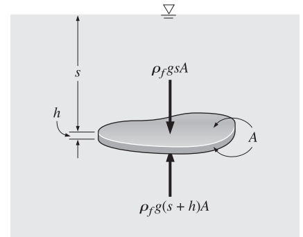
FIGURA 3-37 Placa plana de espesor uniforme h sumergida en un líquido, paralela a la superficie libre.
