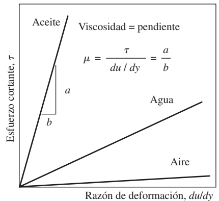
FIGURA 2-13 La razón de deformación (gradiente de velocidad) de un fluido newtoniano es proporcional al esfuerzo cortante, y la constante de proporcionalidad es la viscosidad.
