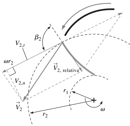
FIGURA 14-95 Vectores de velocidad relativa y absoluta y configuración geométrica para el radio externo del rotor de una turbina Francis. Los vectores de velocidad absoluta están en negritas.
