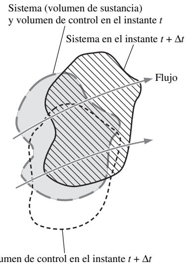
FIGURA 4-62 El volumen de sustancia (sistema) y el volumen de control ocupan el mismo espacio en el instante t (el área sombreada), pero se mueven y se deforman de manera diferente. En un instante ulterior no son coincidentes.
