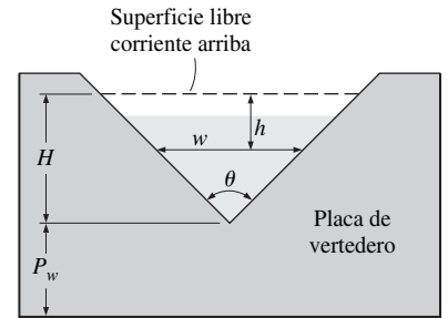
FIGURA 13-44 Geometría de un vertedero triangular (o de forma de “V”) de pared delgada. Esta vista es corriente abajo mirando corriente arriba.
