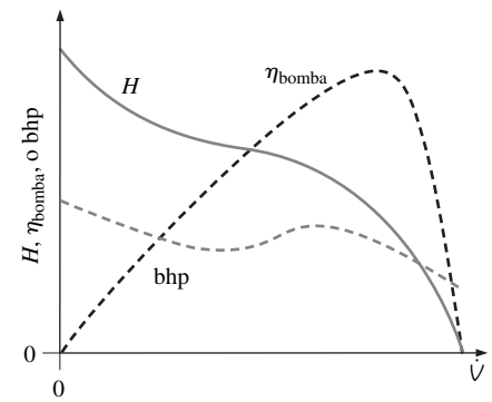
FIGURA 14-60 Curvas de rendimiento típicas de un ventilador de flujo axial con álabes guía.
