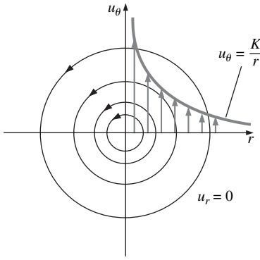
FIGURA 9-47 Líneas de corriente y perfiles de velocidad para un torbellino lineal.
