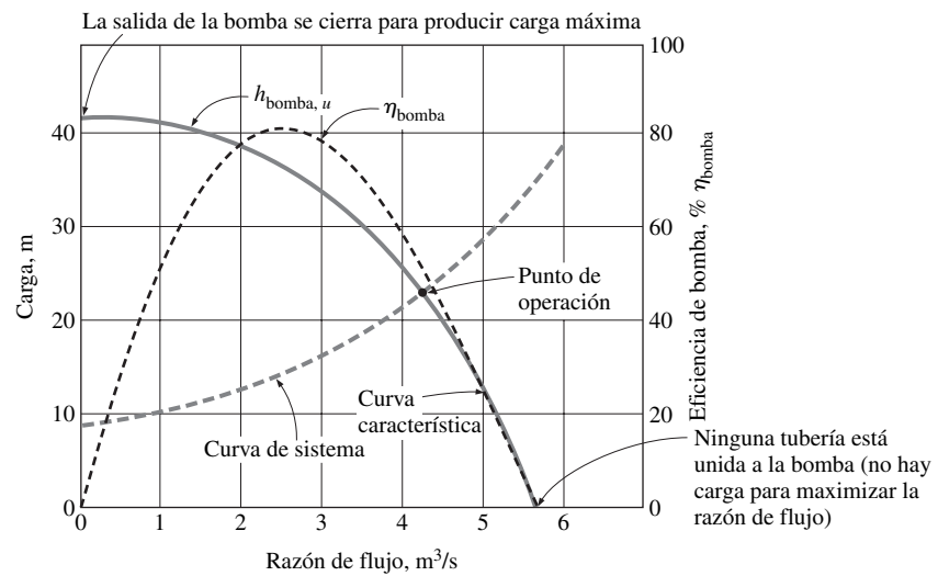
FIGURA 8-46 Curvas características para bombas centrífugas, curva de sistema para un sistema de tuberías y punto de operación.
