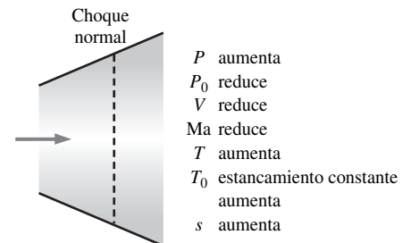
FIGURA 12-32 Variación de las propiedades del flujo a través de un choque normal.
