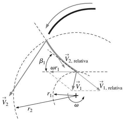
FIGURA 14-96 Vectores de velocidad relativa y absoluta y configuración geométrica para el radio interno de un rotor de una turbina Francis. Los vectores de velocidad absoluta están en negritas.
