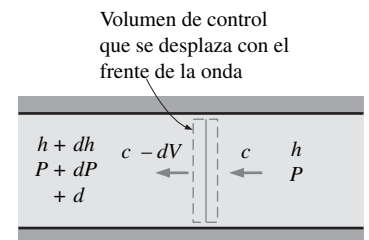
FIGURA 12-8 Volumen de control que se mueve con la pequeña onda de presión en un ducto.
