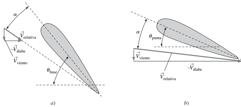
FIGURA 14-51 Cálculo gráfico \vec{V}_{relativa} con dos radios: a) base y b) punta del álabe del rotor que se ilustra en la figura 14-50.
