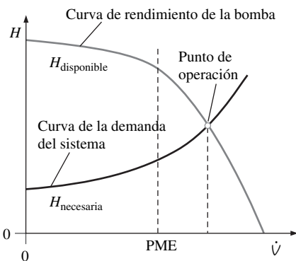
FIGURA 14-9 El punto de operación de un sistema de tuberías se establece como el gasto volumétrico en donde la curva de la demanda del sistema y la curva de rendimiento de la bomba se interceptan.
