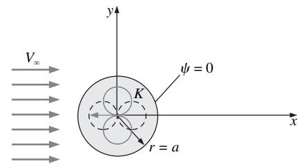
FIGURA 10-60 La superposición de un flujo uniforme y un doblete produce una línea de corriente que es un círculo.
