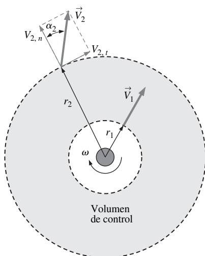
FIGURA 14-38 Volumen de control y vectores de la velocidad absoluta para el soplador centrífugo del Ejemplo 14-5. La vista es a lo largo del eje del soplador.
